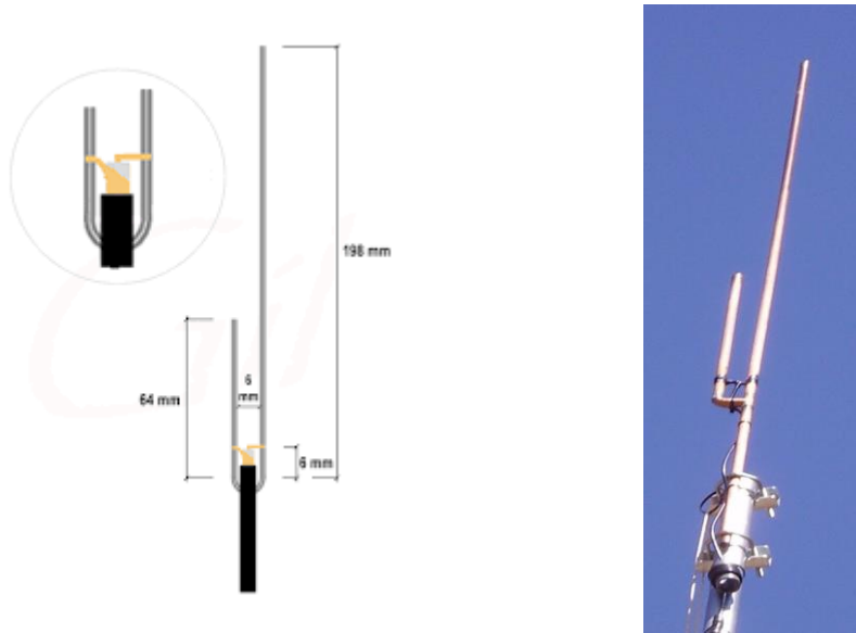
Izq. Esquema teórico de una antena J para la banda de VHF y Dcha. Ejemplo de una antena J ya construida e instalada, similar a la que disfrutó Merche Vidal EB5JDB
