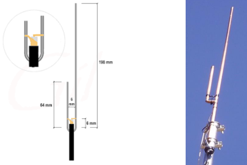
Izq. Esquema teórico de una ante J para la banda de VHF y Dcha . Ejemplo de una antena J ya construida e instalada, similar a la que disfrutó Manolo Peset EB5JDA
