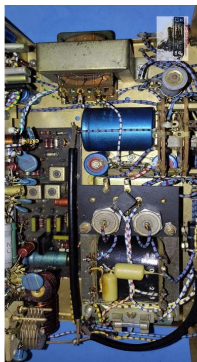
Interior de la emisora de 27 mhz de la marca Luprix, Luis Prieto EA3HX años 60 y 70.
